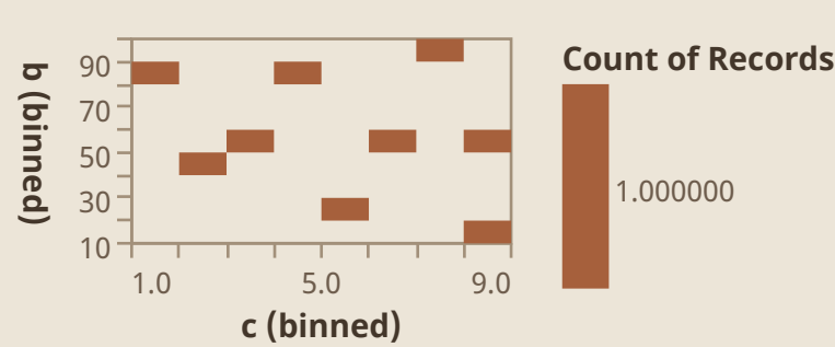
2D-histogrammi · 104 komentoa
