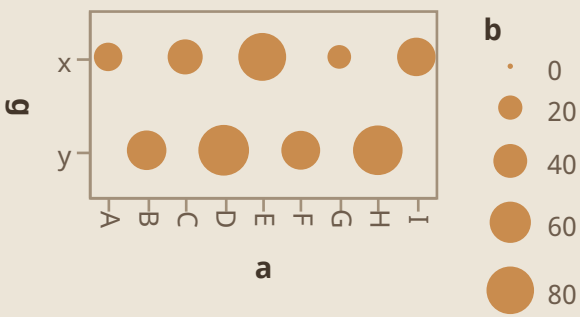
Kuplataulukko · 67 komentoa
