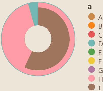
Sädekaavio · 52 komentoa
