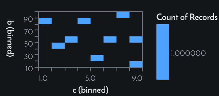
2D-histogrammi · 104 kommentoa
