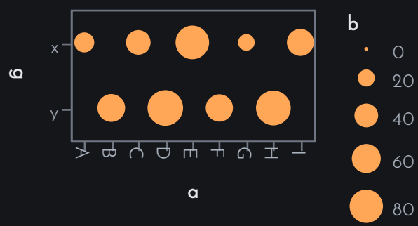
Kuplataulukko · 67 kommentoa
