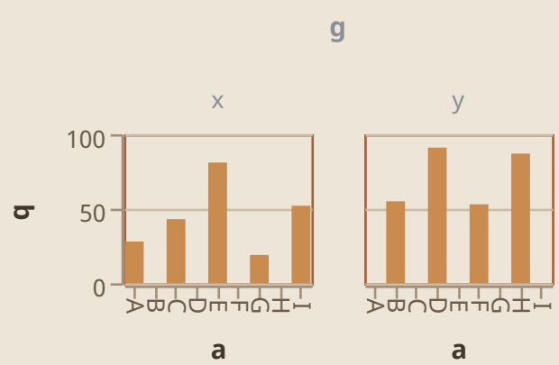
Sarakefasetointi · 102 komentoa
