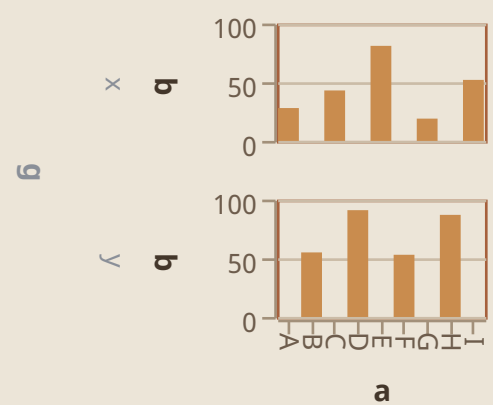
Rivifasetointi · 86 komentoa
