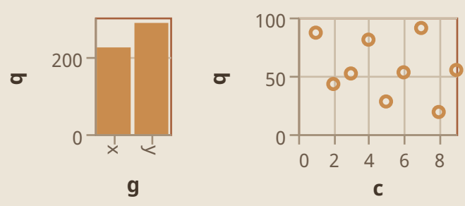
Konkatenaatio · 82 komentoa
