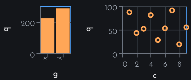
Konkatenaatio · 82 komentoa
