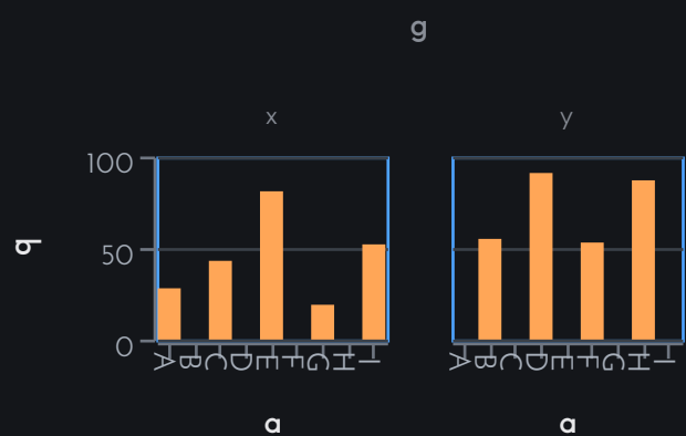
Sarakefasetointi · 102 komentoa
